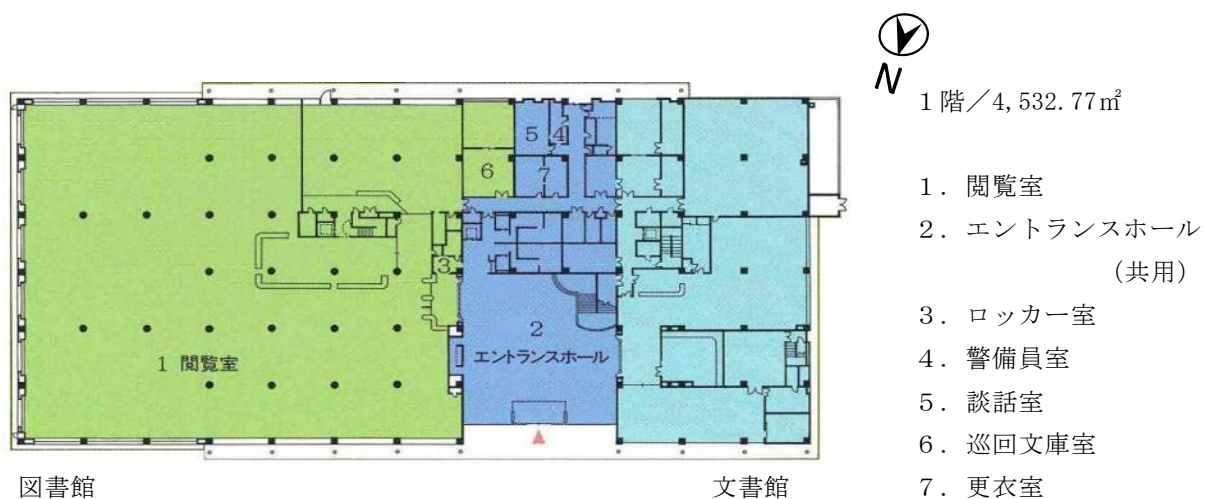
1階平面図
