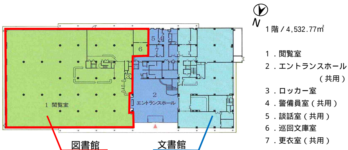
1 階平面図
